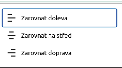
Obr. 42: Možnosti zarovnání
